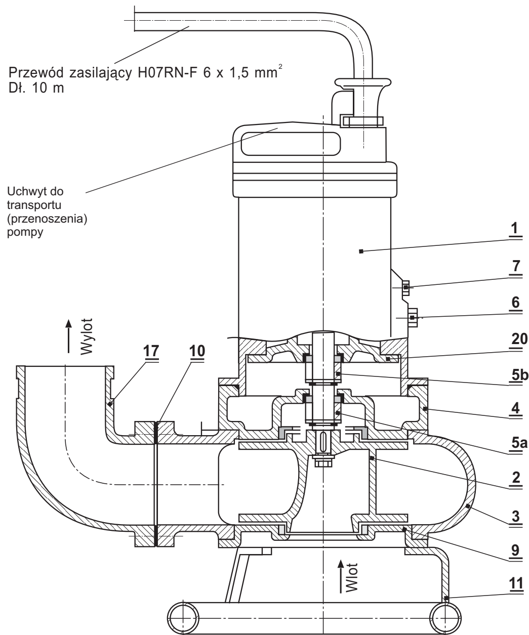
Rys.2z. Budowa pomp typu 100 PZM .../K...-6 (przenośnych - ze stojakiem)
