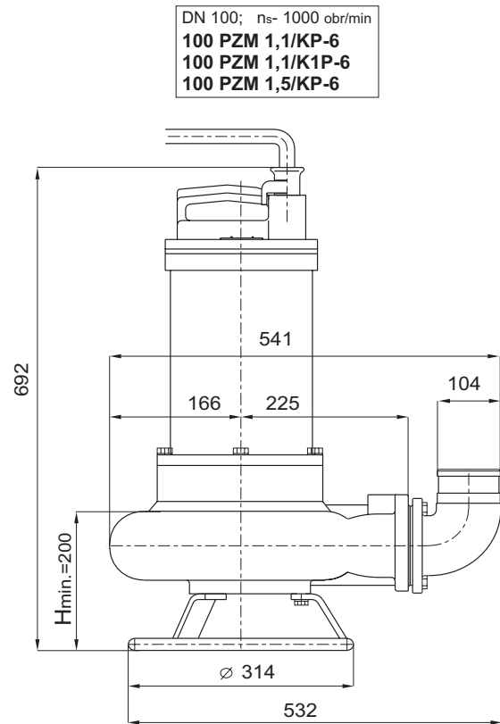
Rys.4z. Wymiary pomp typu 100 PZM .../K...-6 (przenośnych - ze stojakiem)
