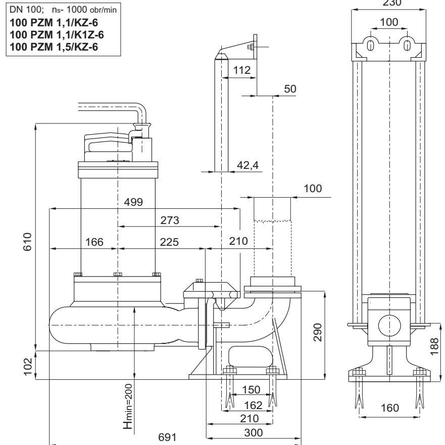
Rys.5z. Wymiary pomp 100 PZM .../K...-6 (stacjonarnych z zaczepem)
