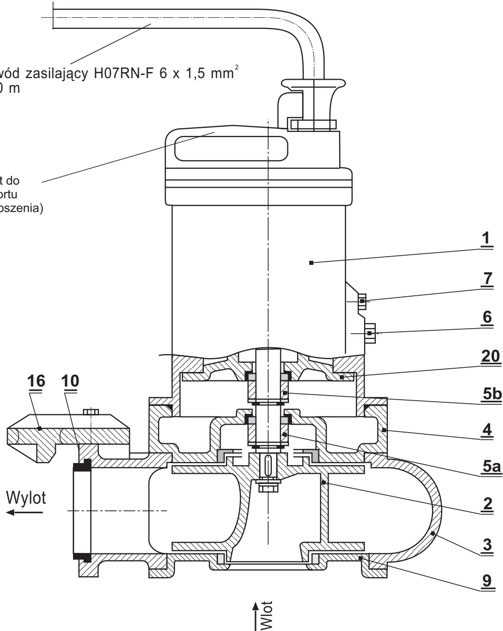
Rys.3z. Budowa pomp typu 100 PZM .../K...-6 (stacjonarnych - z zaczepem)
